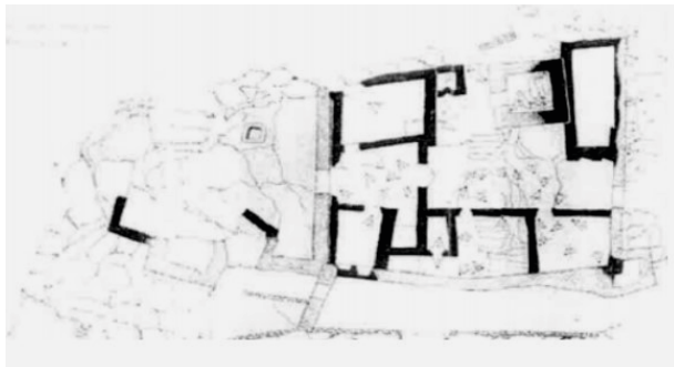
Fig. 4. Rocca di Trevignano: pianta delle murature – in nero le più tarde – (di F. Mezzetti) (da C. PISU, Trevignano Romano: ipotesi d'individuazione del sito di età pre-romana , in "Italia Antiqua" 2012, fig. 6)
